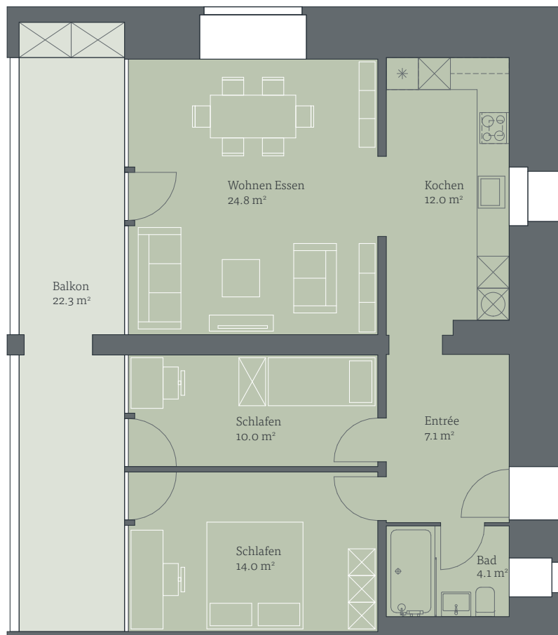
1. Obergeschoss
